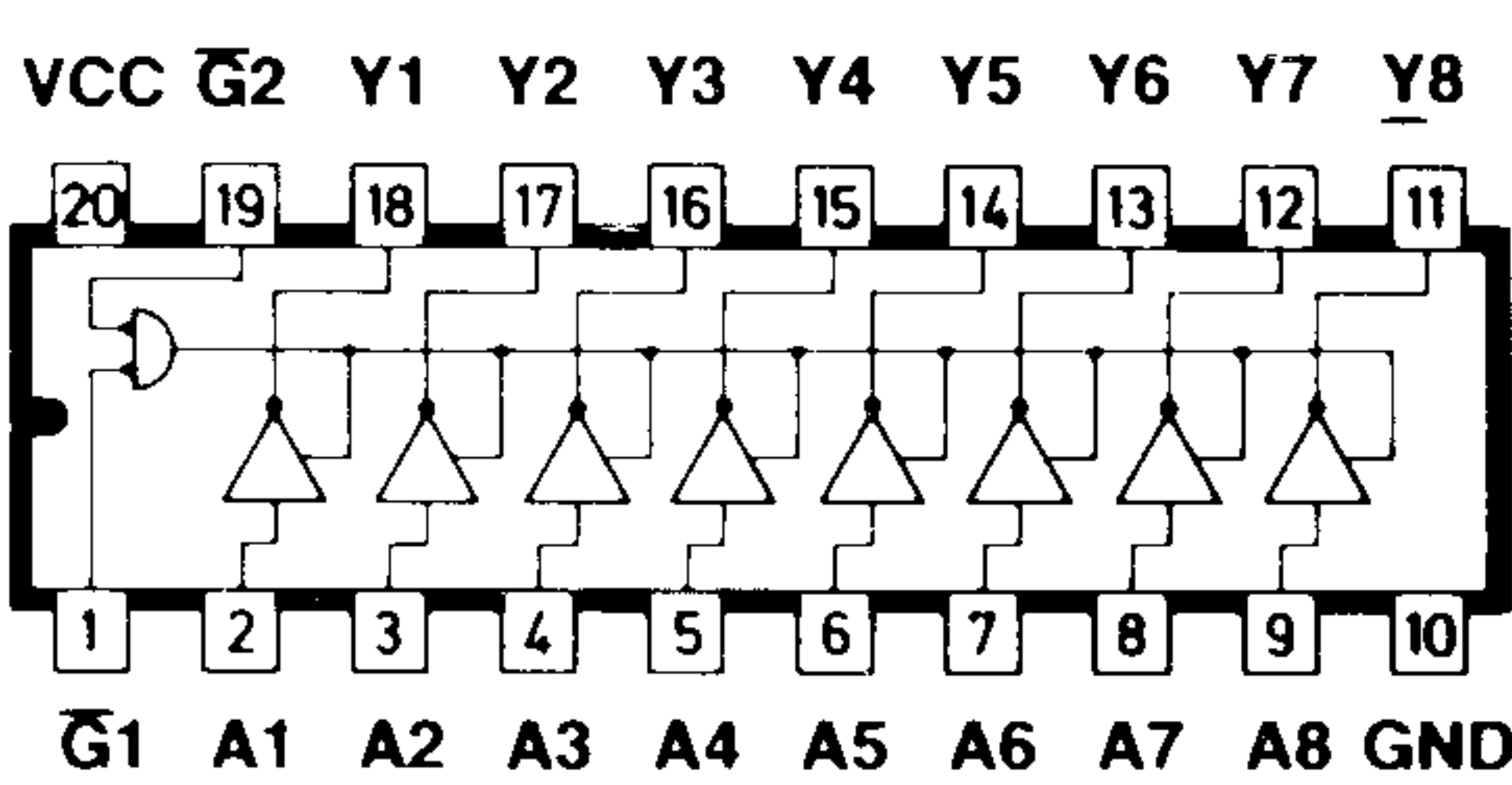
SN74LS541
