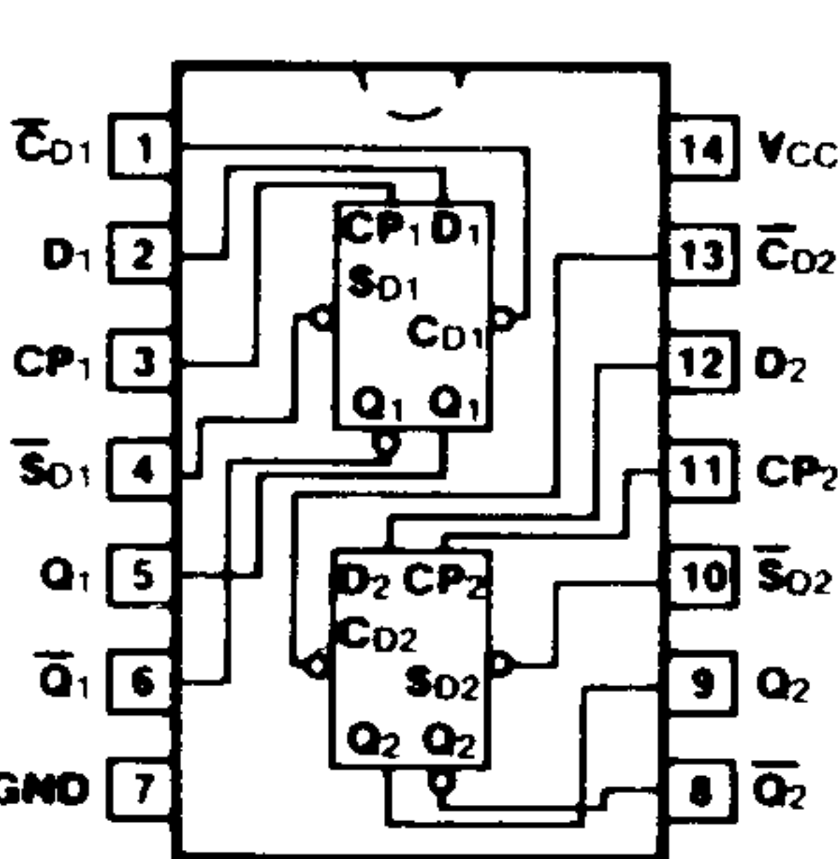
74F74
