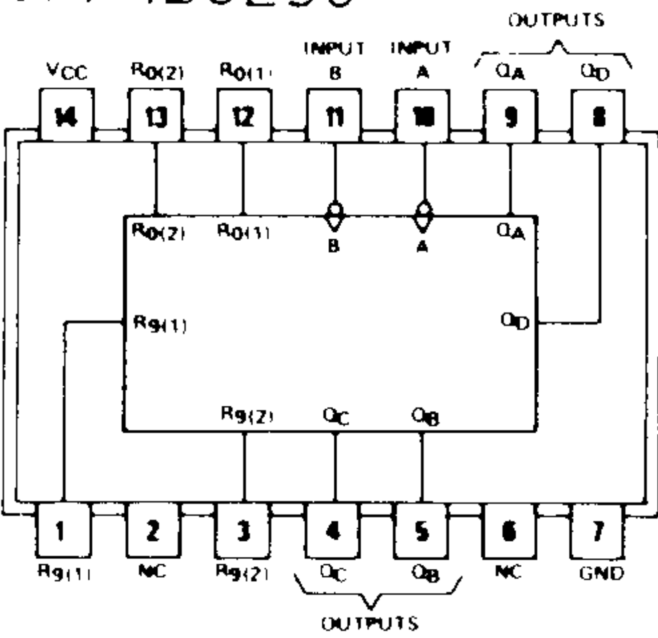
SN74LS290
