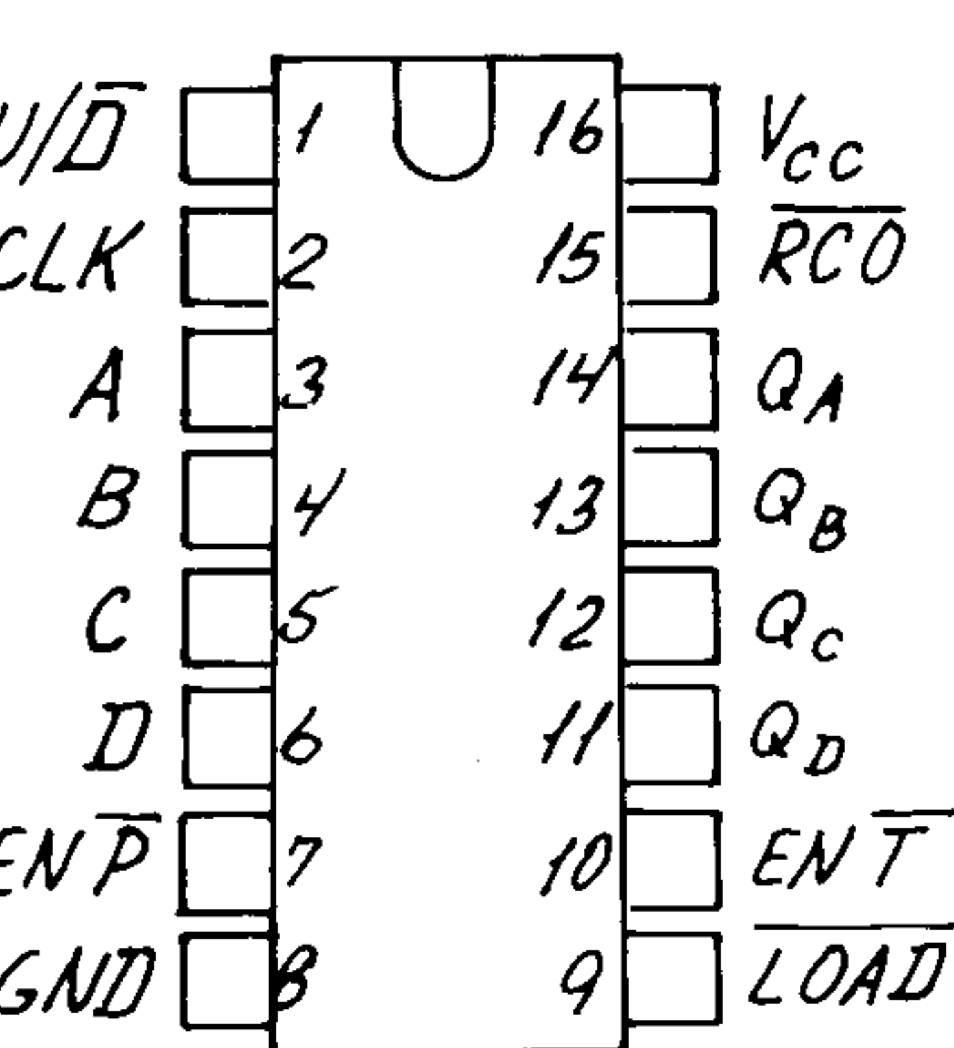
SN74LS669N
