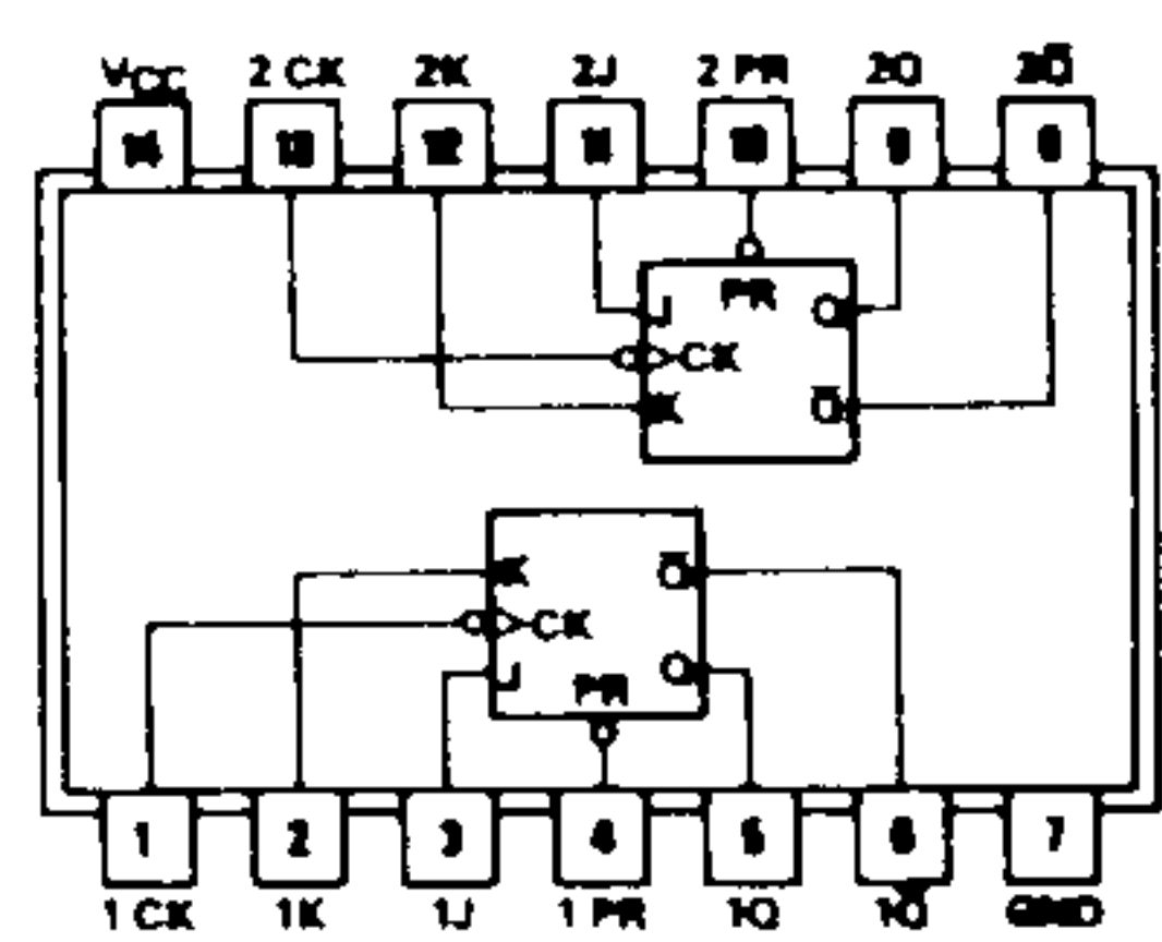
SN74LS113AN
