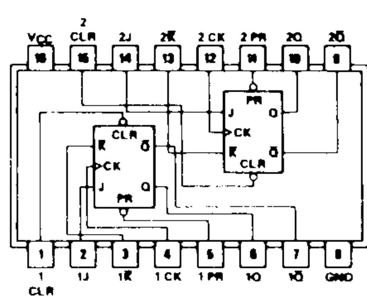
SN74LS109AN
