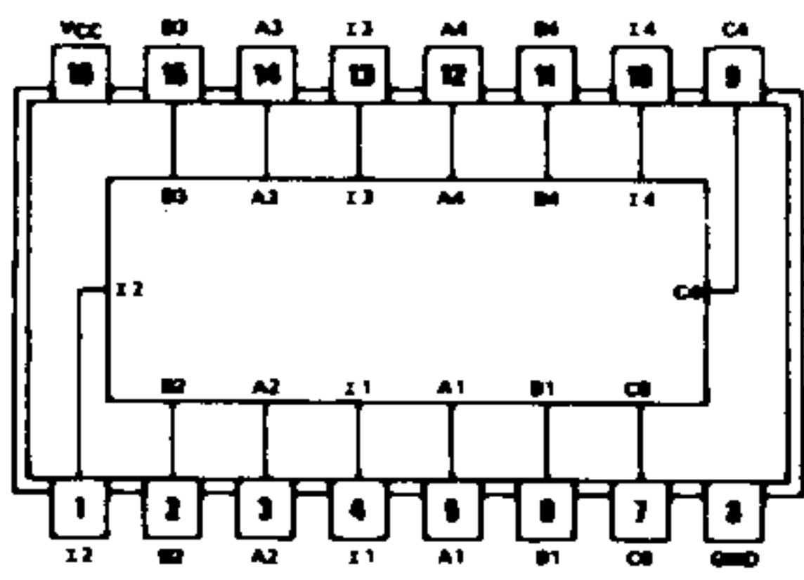
SN74LS283N
