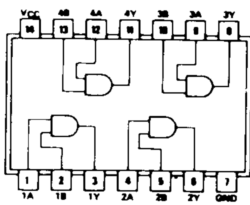
SN74S08N
