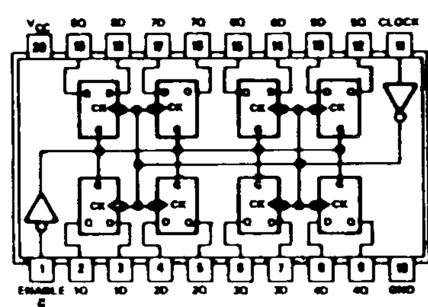
SN74LS377N
